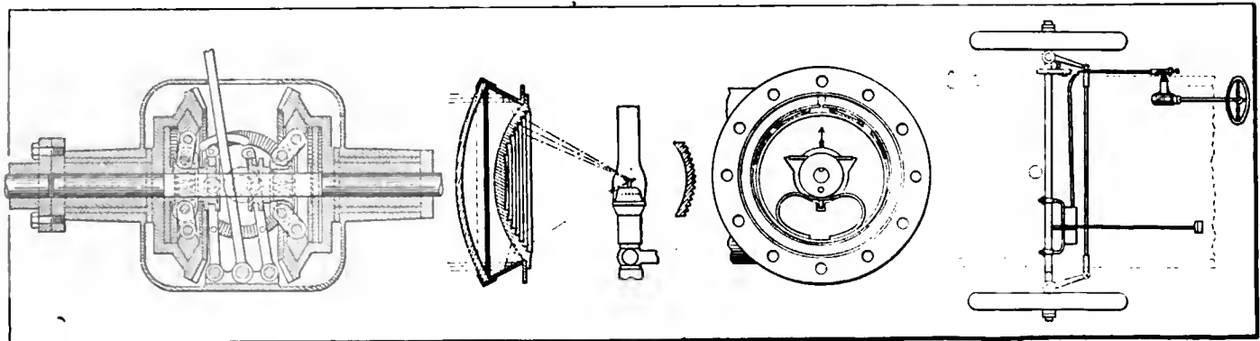
Fig. 4—Benton steering gear
